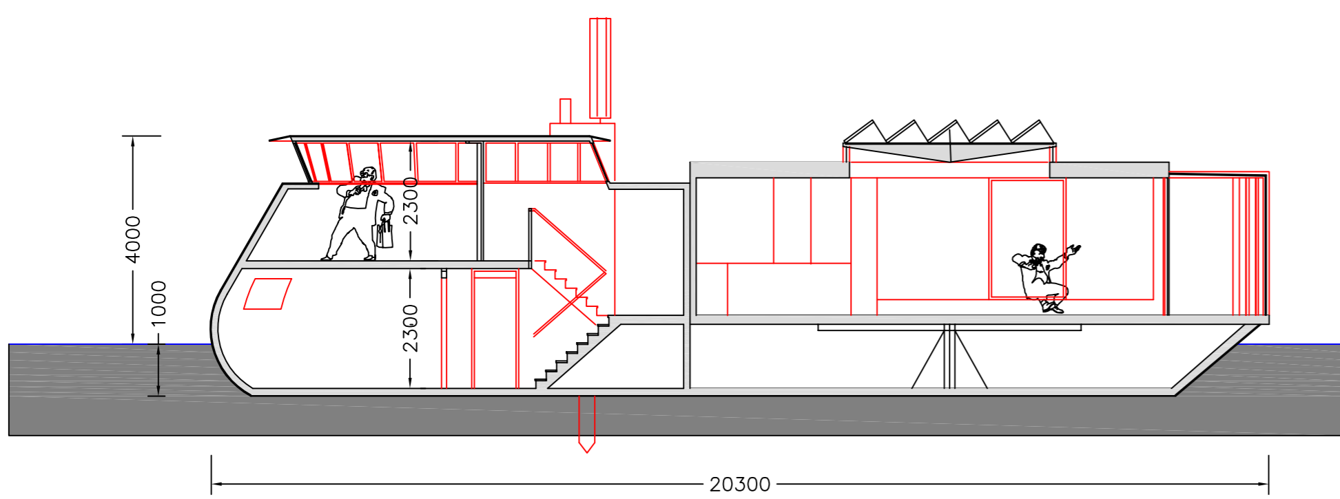
doorsnede
