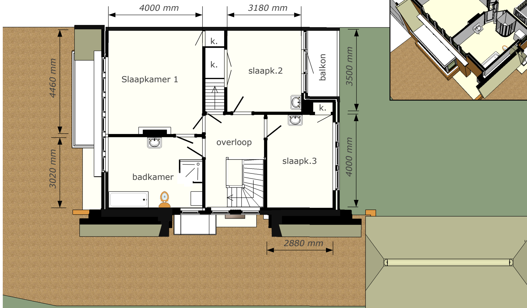
Verdieping
