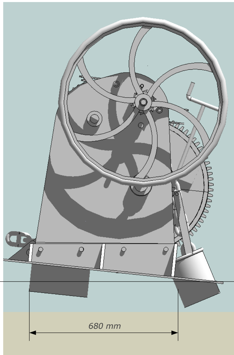
Zijaanzicht
