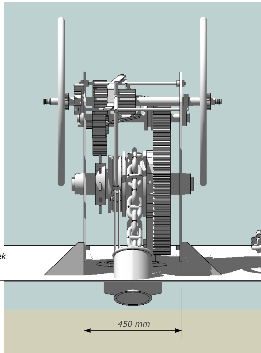
Vooraanzicht
