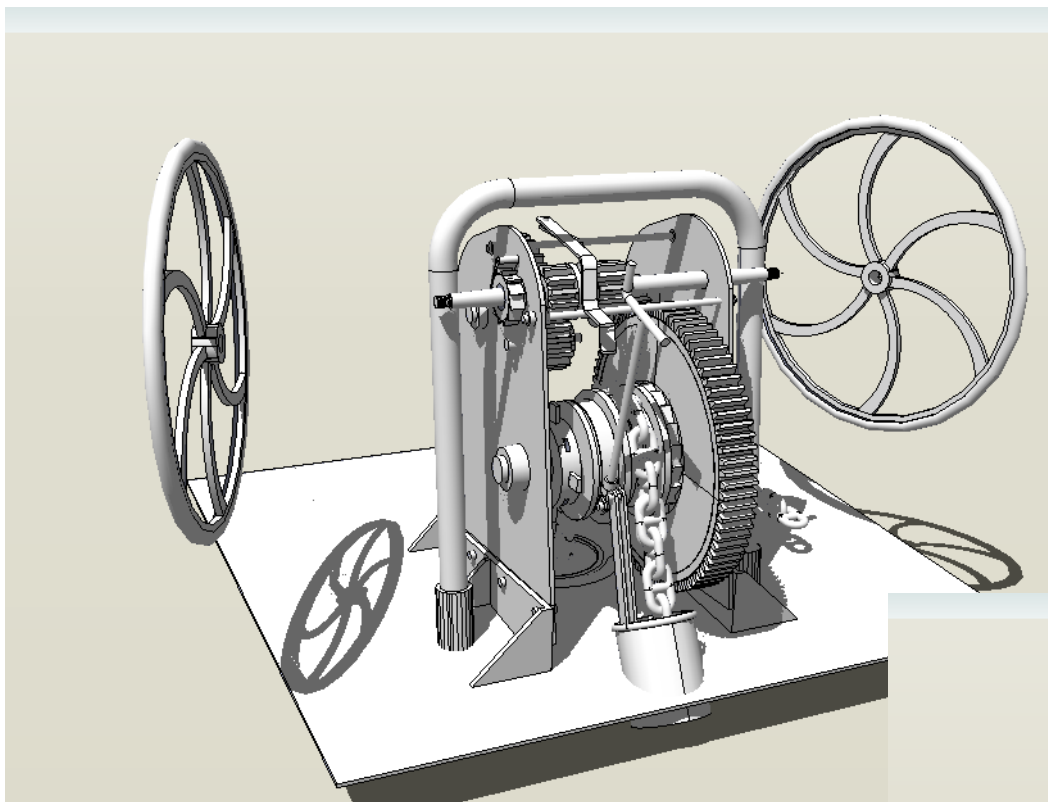
vaarstand, beschermbuis gemonteerd jaagwielen met wartels tegen binnenkant verschansing
