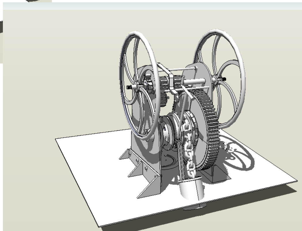
anker inhalen, beschermbuis verwijderd, jaagwielen gemonteerd
